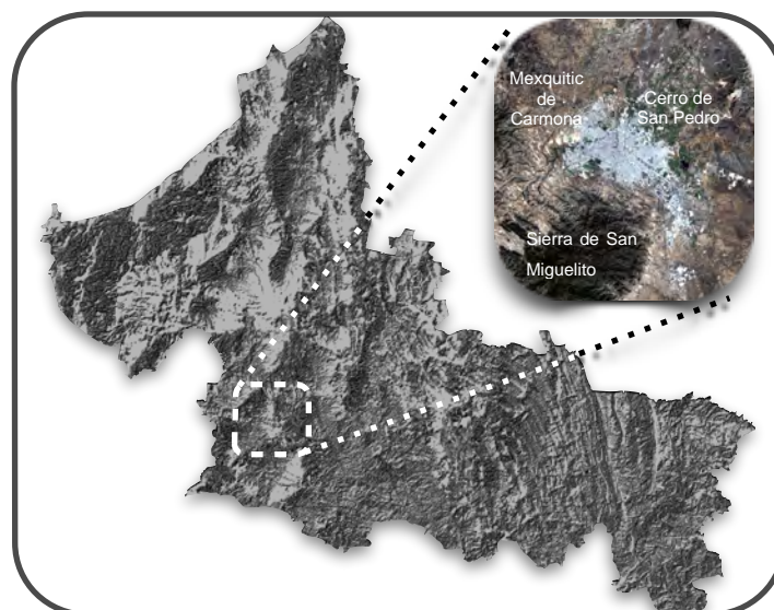
FIGURA 1.1.- UBICACIÓN DEL ÁREA DE ESTUDIO EN EL VALLE DE SAN LUIS POTOSÍ.
