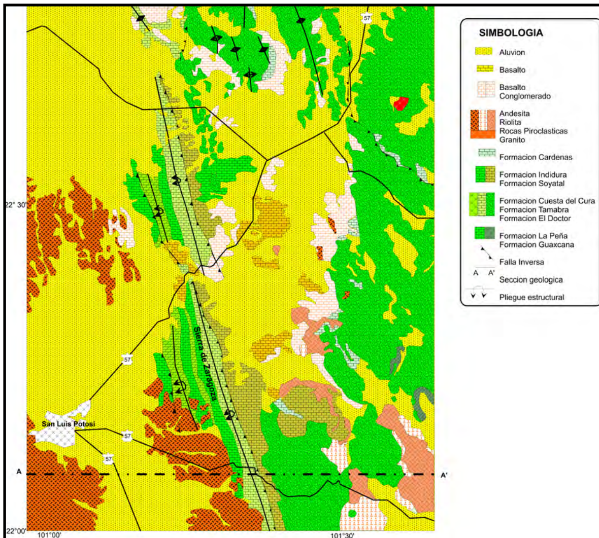
FIGURA 1.3.- GEOLOGÍA REGIONAL DE SAN LUIS POTOSÍ.
