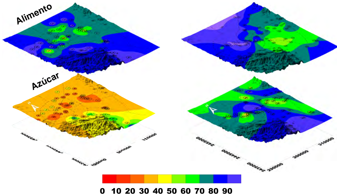
FIGURA 4.7.- MAPA DE DISTRIBUCIÓN DE LA CALIDAD DEL AGUA PARA LA INDUSTRIA DE LA BEBIDA Y ALIMENTOS.
