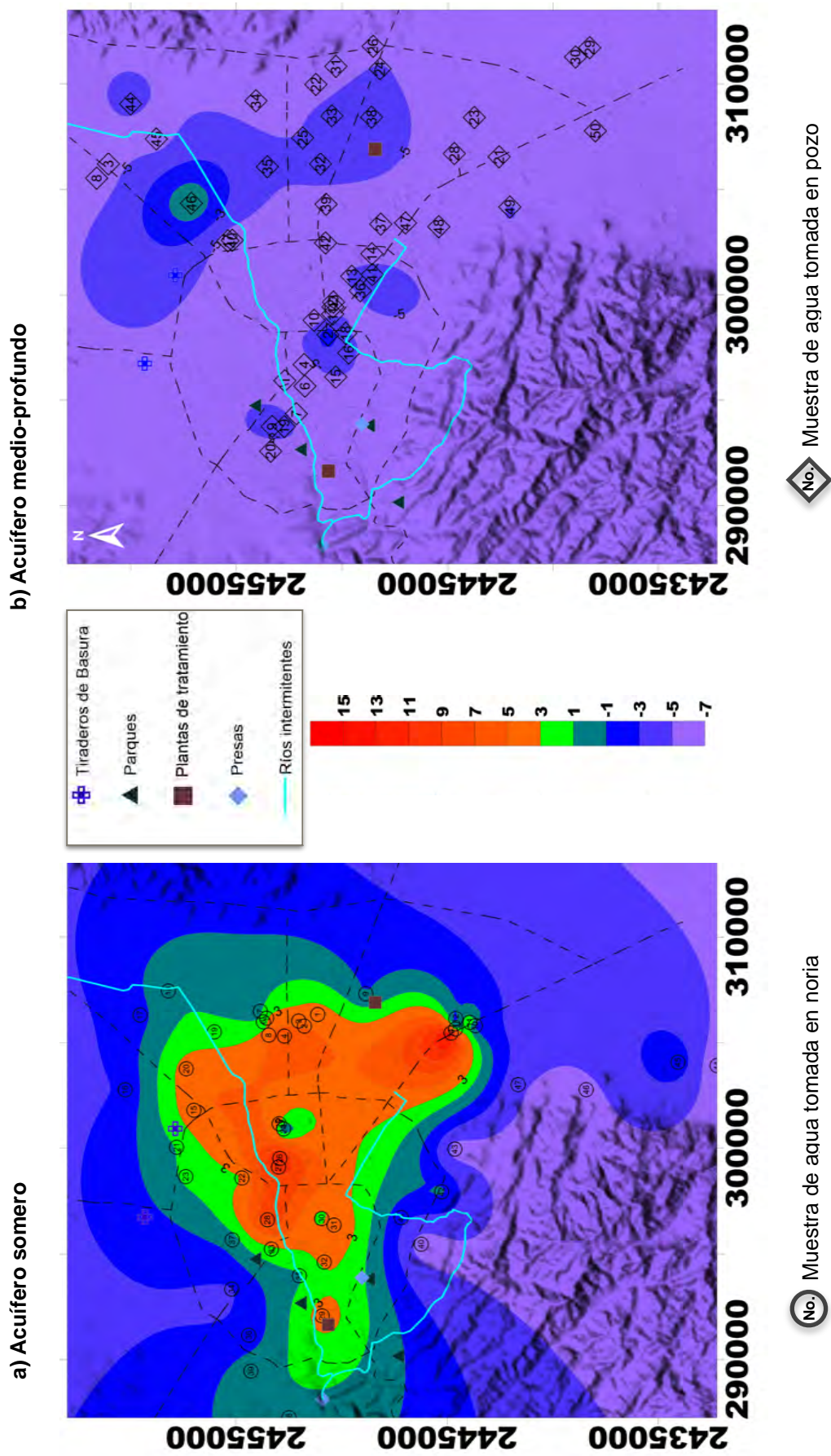
FIGURA 4.2.- DISTRIBUCIÓN ESPACIAL DEL ÍNDICE DE CONTAMINACIÓN (ICON).
