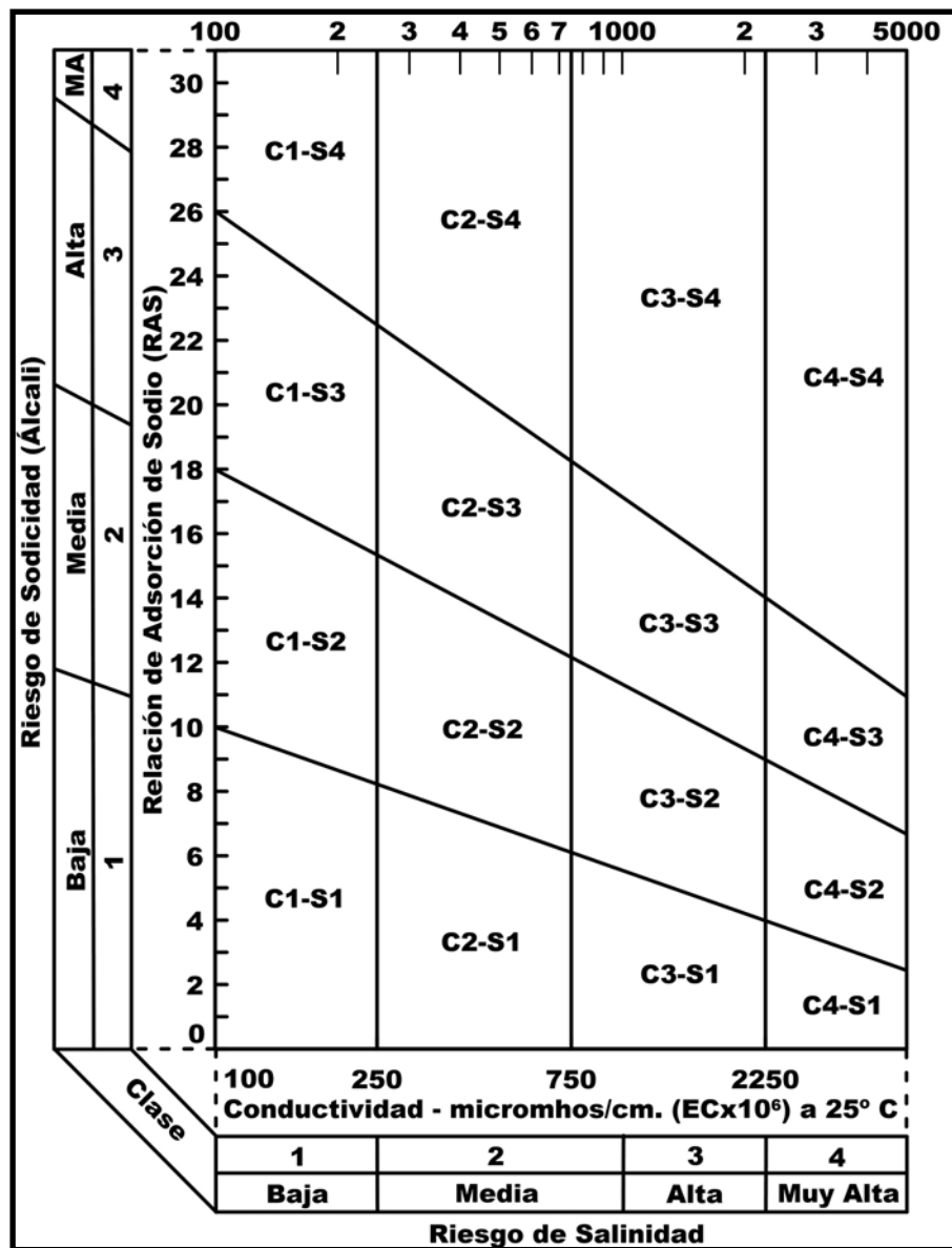
GRÁFICO 3.1.- CLASIFICACIÓN DE SALINIDAD DE ESTADOS UNIDOS DE MANANTIALES Y AGUAS SUBTERRÁNEAS PARA RIEGO (RICHARDS, 1954).
