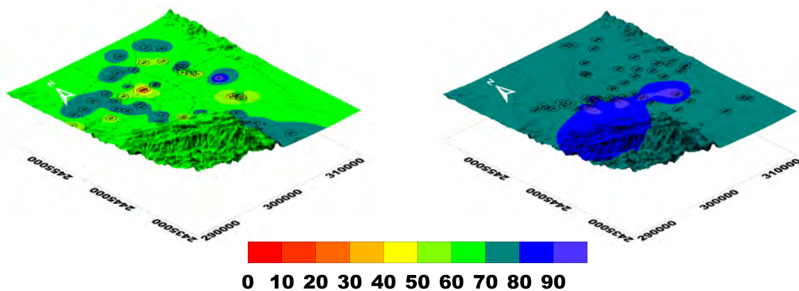
FIGURA 4.6.- MAPA DE DISTRIBUCIÓN DE LA CALIDAD DEL AGUA PARA LA INDUSTRIA DE HIERRO Y ACERO.
