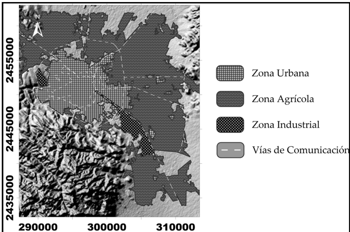
FIGURA 1.2.- USOS DE SUELO EN EL VALLE DE SAN LUIS POTOSÍ
