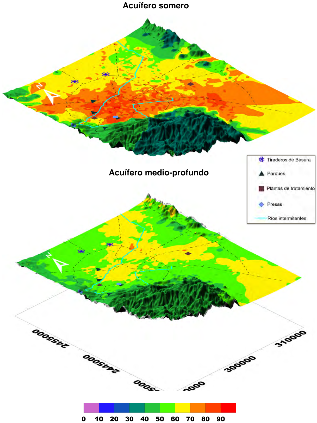
FIGURA 4.10.- DISTRIBUCIÓN ESPACIAL DEL ÍNDICE DE VULNERABILIDAD ACUÍFERA DRASTIC NORMALIZADO.
